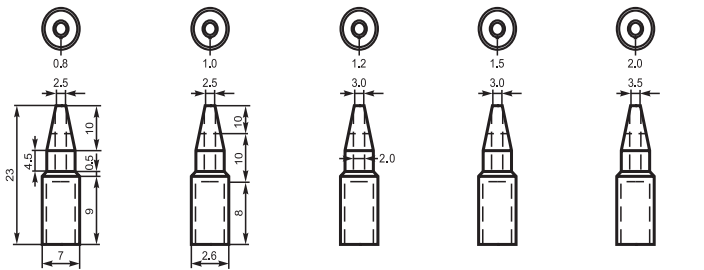
T-928-0.8T T-928-1.0T T-928-1.2T T-928-1.5T T-928-2.0T
